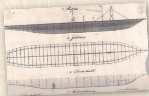
▲ Plan du Franz 1 er , bateau à vapeur mis au point en Autriche.
